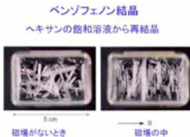
図3 ベンゾフェノン結晶の磁気配向
