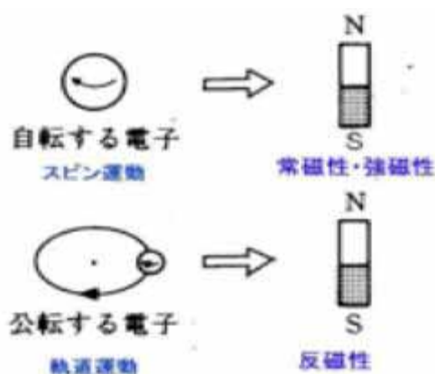
図1 磁性の起源
