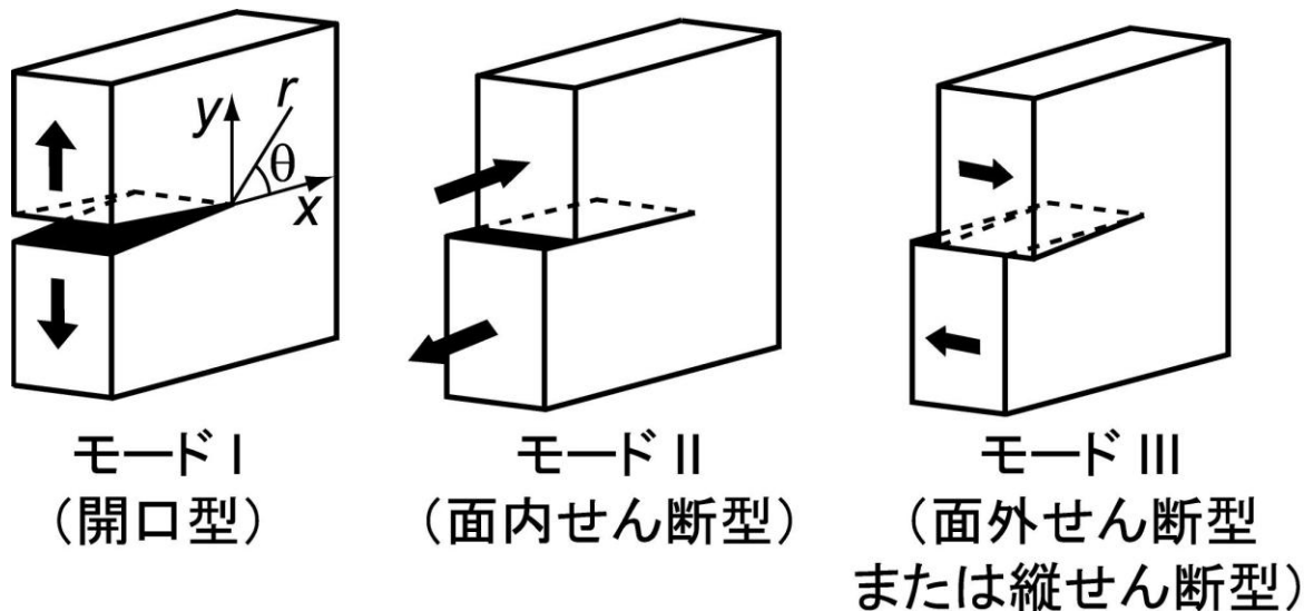
図 2 き裂が伝ばするときの力の加わり方。モード I : 割り箸を割るときのように、上下に引張り力を加える。モード II : トランプを重ねて横にずらすときのように、せん断力を加える。モード III : 「するめ」の入った袋を開けたり、「するめ」そのものを裂いたりするときのように、前後にせん断力を加える。実際には、2つ以上のモードが混じっている場合も多い。
